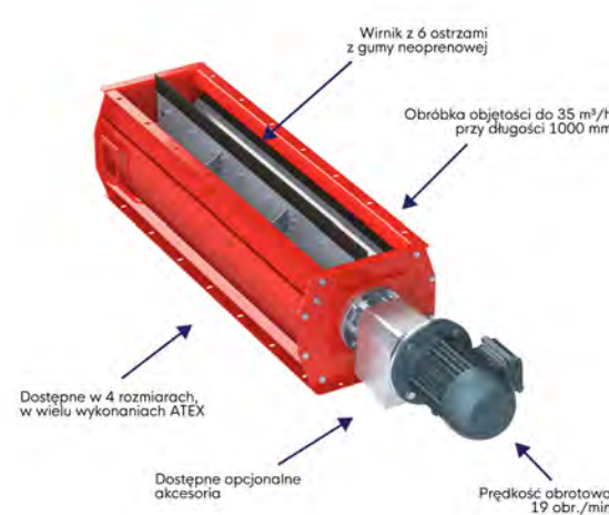
Zawór obrotowy RVA-X
