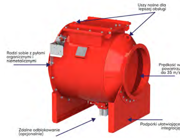
Zawór przeciwwybuchowy BADA-FAB
