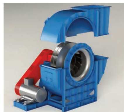
Dviejų dalių korpusas
