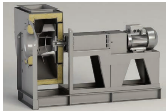
Korpusas su pilna izoliacija kompl. 8
