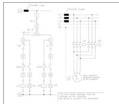
Schéma de raccordement électrique
